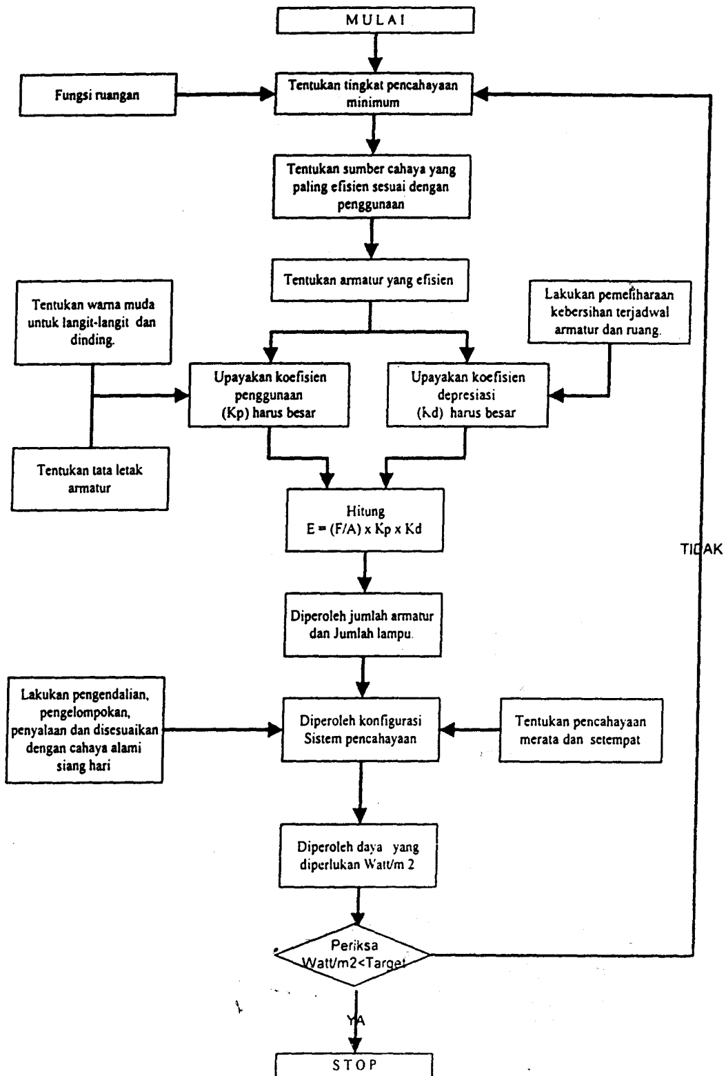
Gambar 1 Prosedur perencanaan teknis sistem pencahayaan buatan
